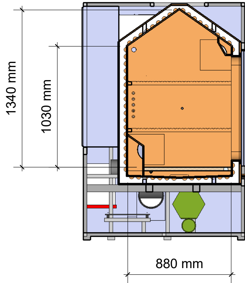
Schnitt A-A
